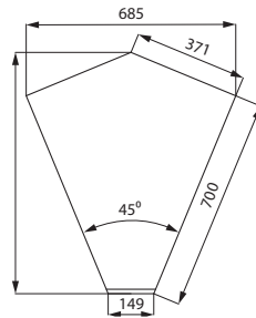
STANOWISKO NAROŻNE WEWNĘTRZNE OTWARTE 45° DM-94973
