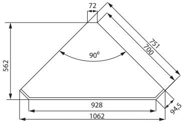
STANOWISKO NAROŻNE ZEWNĘTRZNE OTWARTE 90° DM-94972-0
