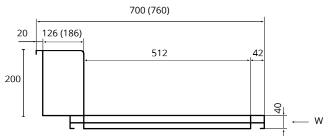
Standardbefestigung an Beladetischen für Geschirrspüler: DM-3266, DM-3268, DM-3257, DM-3247
