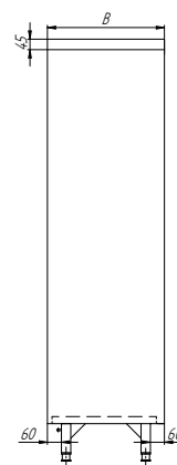
DURCHREICHESCHRANK MIT SCHIEBETÜREN DM-3309
