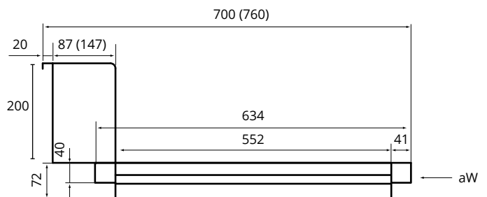
Standardbefestigung an Rollenbeladetischen für Geschirrspüler: DM-3275, DM-3276
