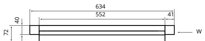
Standardbefestigung an Rollenentladetischen für Geschirrspüler: DM-3277, DM-3278
