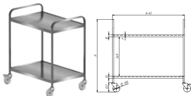
KELLNERWAGEN ZUM ZUSAMMENSCHRAUBEN MIT 2 FACHBÖDEN
