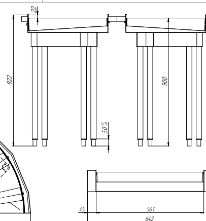
90°-ROLLENECKTISCH FÜR GESCHIRRSPÜLER MIT MANUELLER BESCHICKUNG DMTTAAR90C
