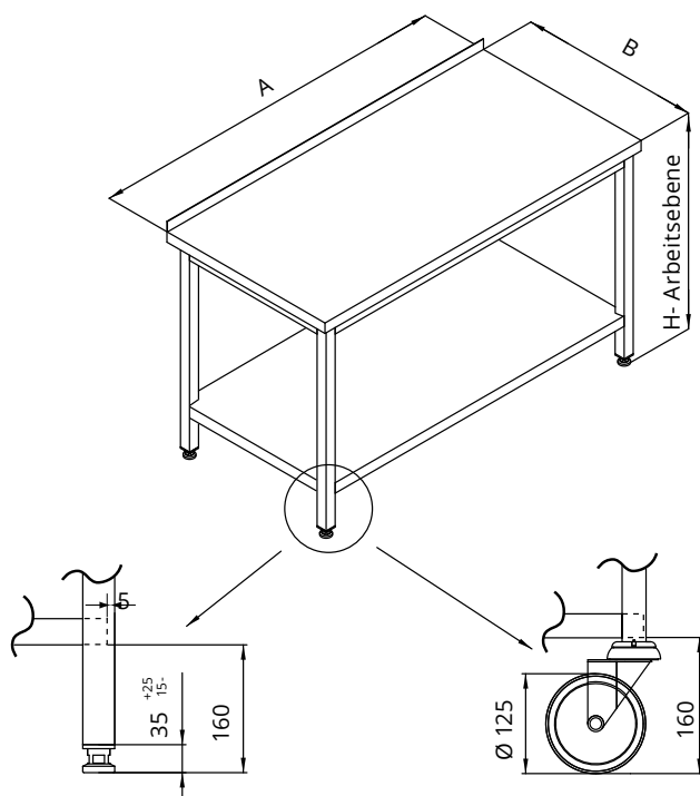
stationäre Ausführung
