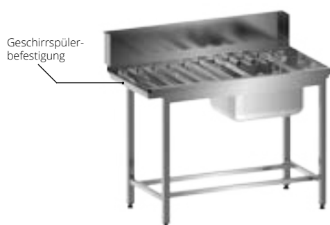
ROLLENBELADETISCH MIT SPÜLBECKEN DM-3276
