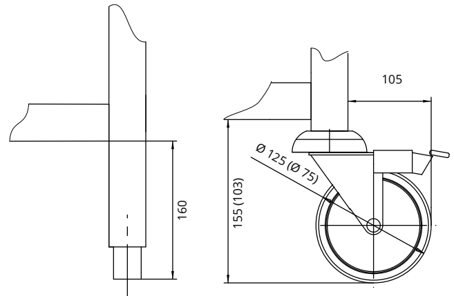
stationäre Ausführung
