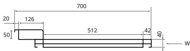
Standardbefestigung an Entladetischen für Geschirrspüler: DM-3265, DM-3248
