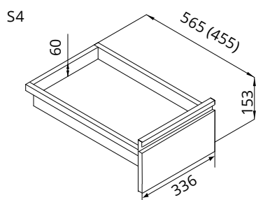
Schubladen S2, S3, S4 (eingebaut in Schränke der Länge A = 400 mm)
