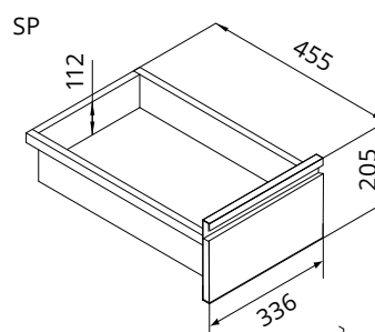
Schubladen SP (Schublade für das Aufhängemodul)
