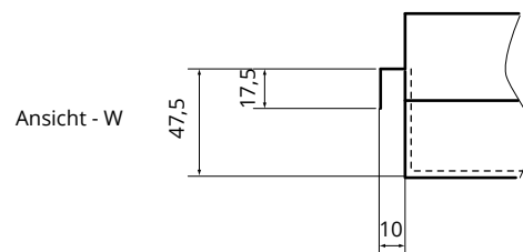
Standardbefestigung an Rollenentladetischen für Geschirrspüler: DM-3277, DM-3278
