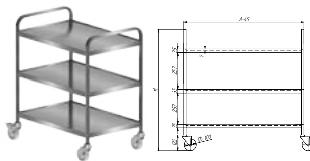
KELLNERWAGEN ZUM ZUSAMMENSCHRAUBEN MIT 3 FACHBÖDEN
