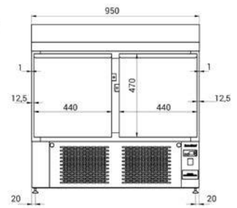
urządzenia z maszynownią w podstawie
