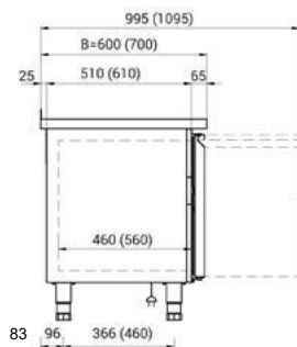
urządzenia z maszynownią z boku
