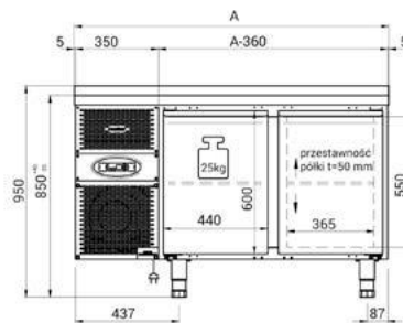
urządzenia z maszynownią z boku
