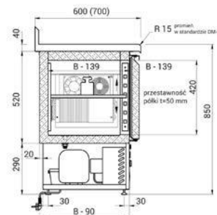
urządzenia z maszynownią w podstawie
