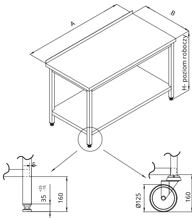
wersja stacjonarna
