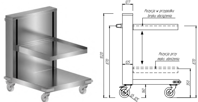
WÓZEK NA TACE Z PODNOSZONĄ PLATFORMĄ DM-3417
