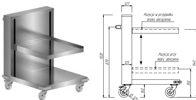
WÓZEK NA KOSZE Z PODNOSZONĄ PLATFORMĄ DM-3416
