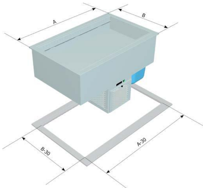
Umieszczenie wanny chłodniczej w płycie
