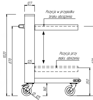
WÓZEK NA TACE Z PODNOSZONĄ PLATFORMĄ DM-3417
