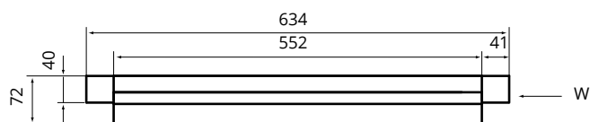
Zaczepek standardowy w stołach wyładowczych rolkowych do zmywarek: DM-3277, DM-3278
